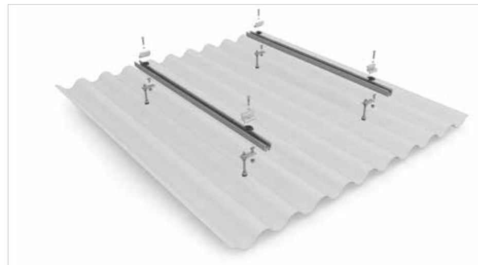
Sistem diagramă descompusă
